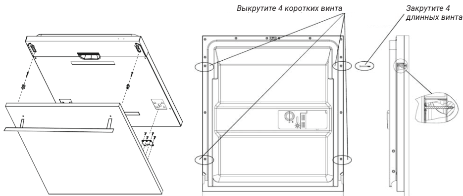
Рис. 4 Установка внешней панели
