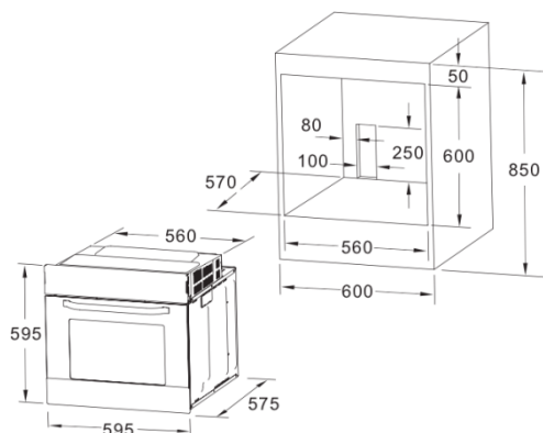
Размеры прибора и требуемой ниши для встраивания
