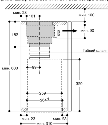
Верхний шкаф с AC 200 и AA 211 812, поперечный разрез
