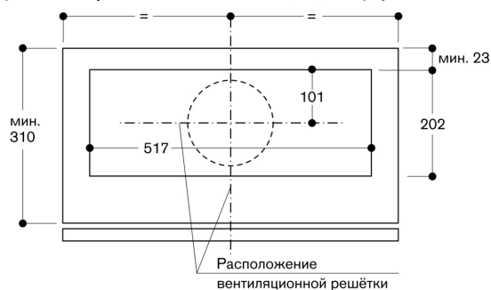
Верхний шкаф с AC 200 и AA 211 812, вид сверху
