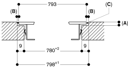
A: 6,5 +0,5 B: 2,5 C: Заполнение силиконом Размеры в мм
