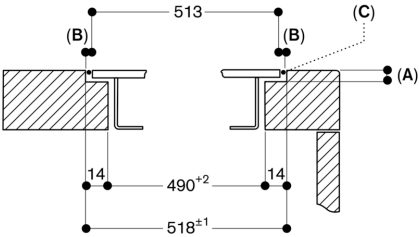
A: 6,5 +0,5 B: 2,5 C: Заполнение силиконом Размеры в мм
