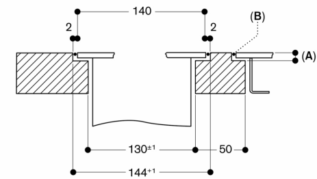
Поперечное сечение
