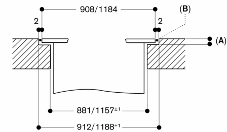
Продольное сечение
