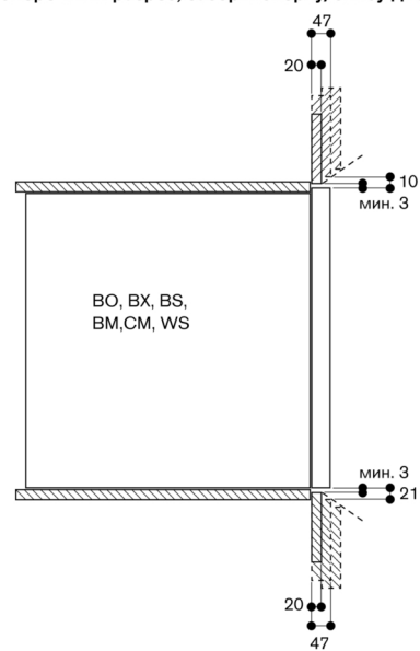
Поперечный разрез, зазоры сверху/снизу дверцы
