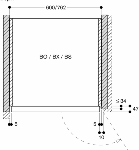
Поперечное сечение воздухозаборного отверстия по краям двери
