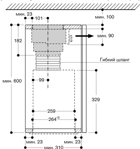
Верхний шкаф с AC 200 и AA 211 812, поперечный разрез
