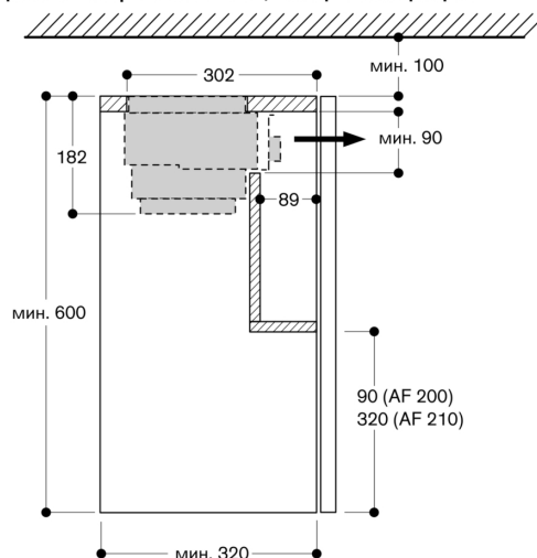
Верхний шкаф с AA 211 812, поперечный разрез
