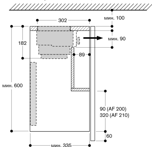
Верхний шкаф, поперечный разрез с AA 211 812 и телескопические рамы AA 210 490/460
