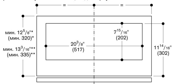
Верхний шкаф с AA 211 812, вид сверху
