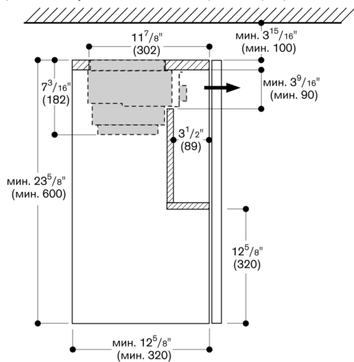
Верхний шкаф с AA 211 812, поперечный разрез
