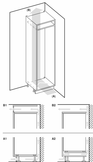
A: Air inlet ≥ 200 cm²; ventilation options A1 or A2 B: Air outlet ≥ 200 cm²; ventilation options B1 or B2
