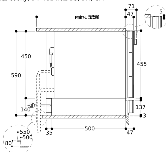
Вид сбоку, DV 461 под BS, BM, CM
