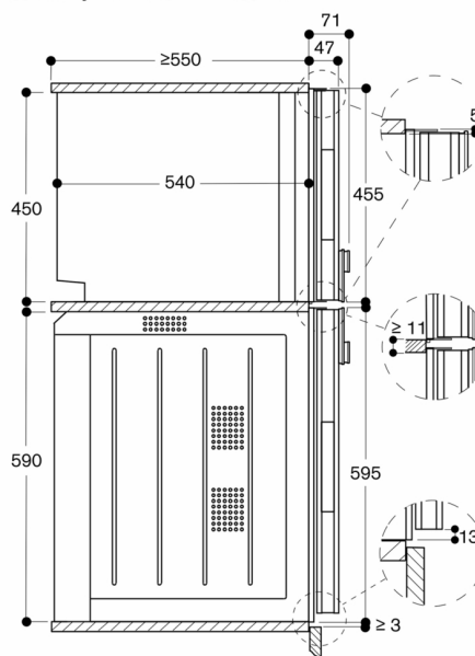
Вид сбоку BS 454/455 над BO
