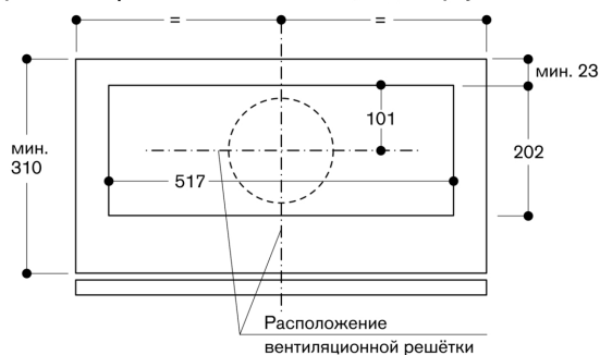
Верхний шкаф с AC 200 и AA 211 812, вид сверху
